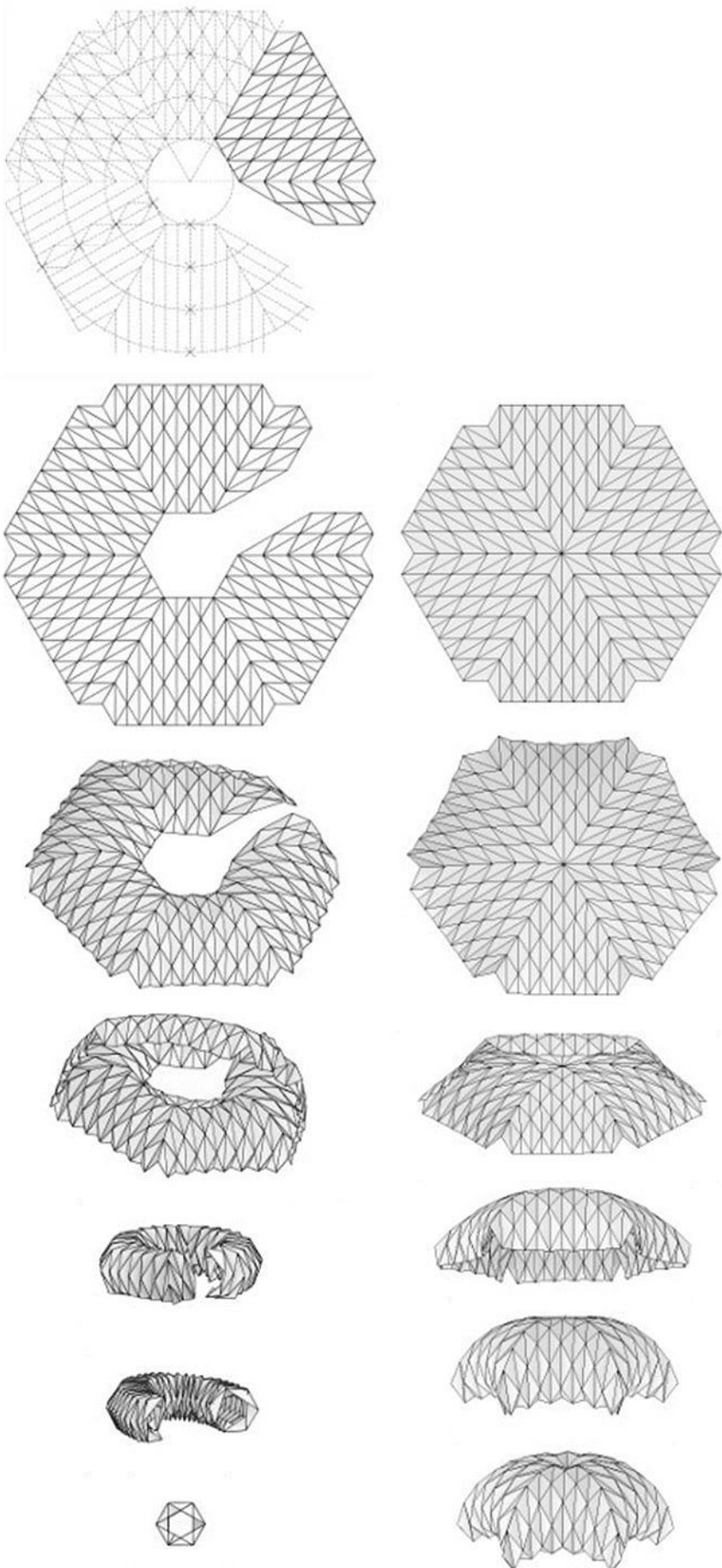
115. Yoshimura Hexagonal Polar Autor Pablo de Souza, 2012. Simulaciones realizadas con el programa Rigid Origami de Tomohiro Tachi.
