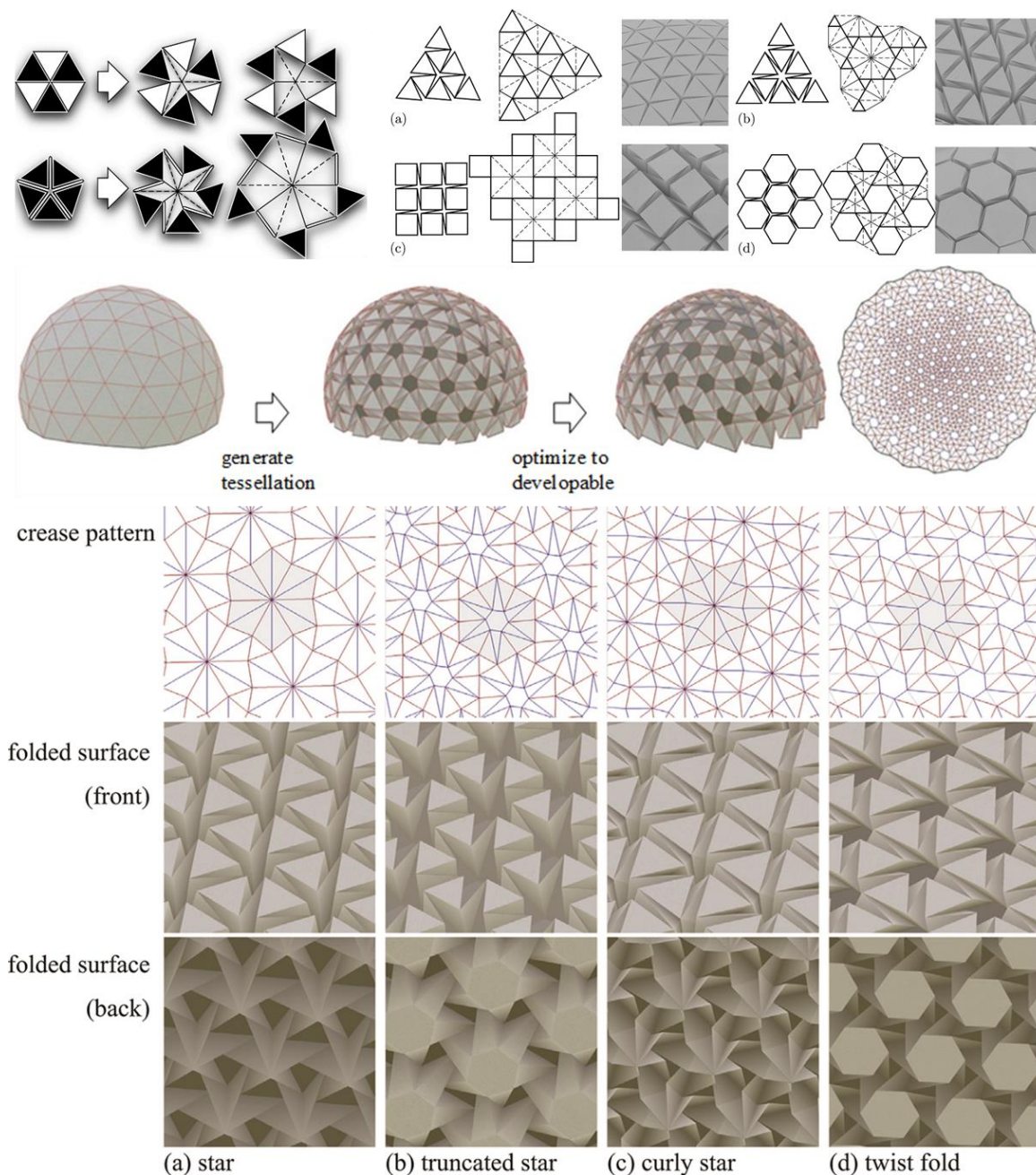
149. Variaciones de teselaciones de Resch realizadas por Tachi
