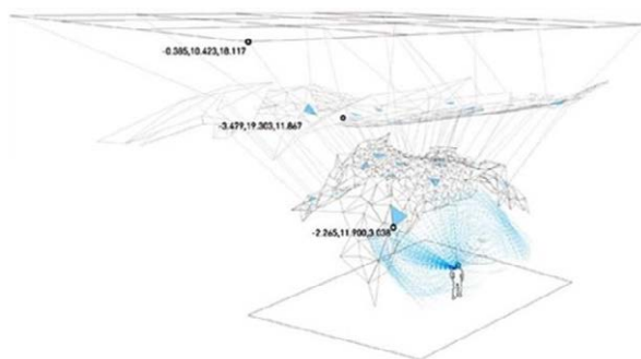
152. Sistema de monitorización, Resonant Chamber, RVTR, 2012.
