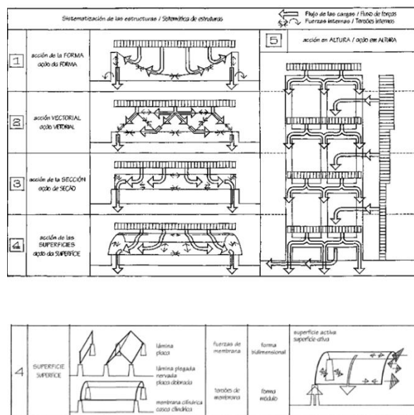
184. Sistemas de Estructuras. Engels 1964 Portada y diagramas de cargas o fuerzas sobre el sistema de clasificación y sistematización de las estructuras
